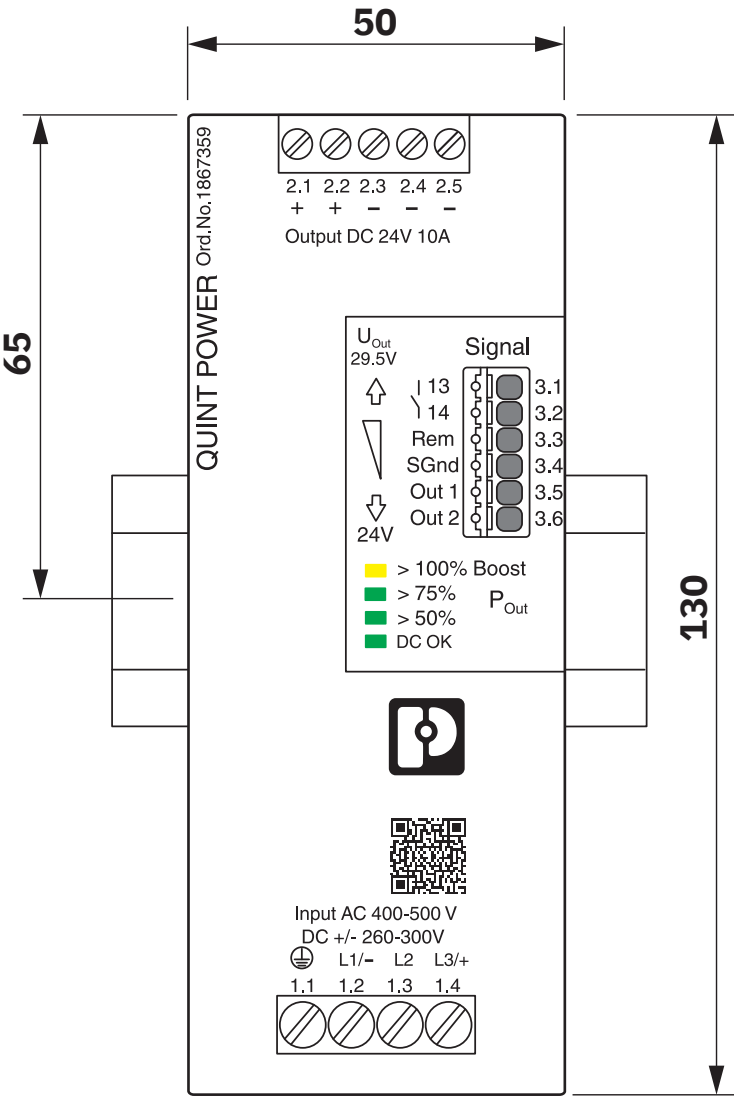
Rysunek wymiarowy
